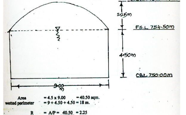
बोगद्याचे रेखांकन
